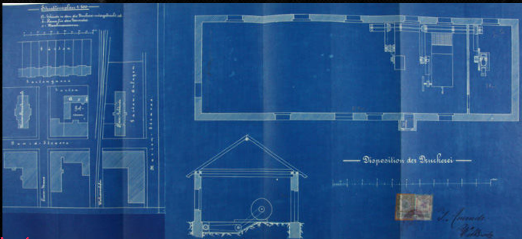
Dispoziční řešení tiskárny, přestěhované do dvorní části domu na dnešní ulici Jeremenkově, rok 1903
