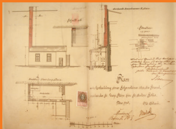
Plán stavby komínu pekařské dílny Antona Polkeho na rohu ulic Zámecké a Dlouhé, 1893
