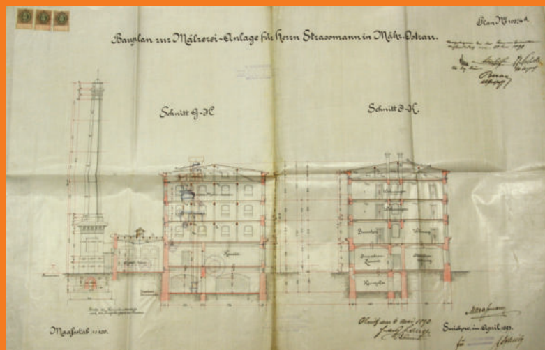
Plán stavby parostrojní sladovny M. Strassmanna na Fifejdách, 1893
