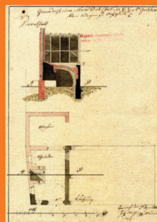
Plán kovářské dílny Johana Grubera z roku 1820 při maloměstském domě č. 7 na Vitkovickém předměstí v Moravské Ostravě
