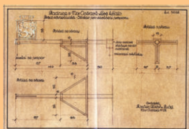
Schéma praporevého stožáru firmy Franta Anýž
