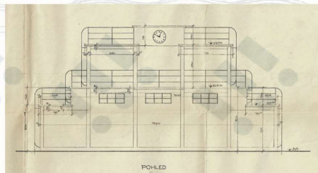
Nejpokrokovějším prvkem ostravského koupaliště bylo spojení filtrační stanice se skokanskou věží, která přiléhala k bazénu ze západní strany. Odvážlivci si mohli skočit do vody ze dvou úrovní – 3,7 m a 6,2 m (30. léta 20. stol.)
